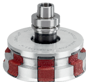
Utensile a levigare per battute
