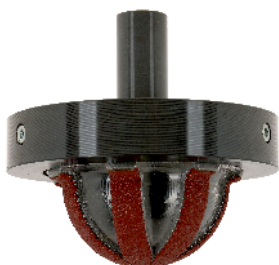
Utensile a levigare per incastri decorativi
